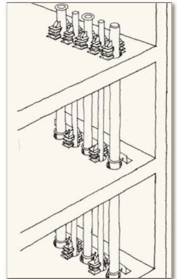
防振固定部
