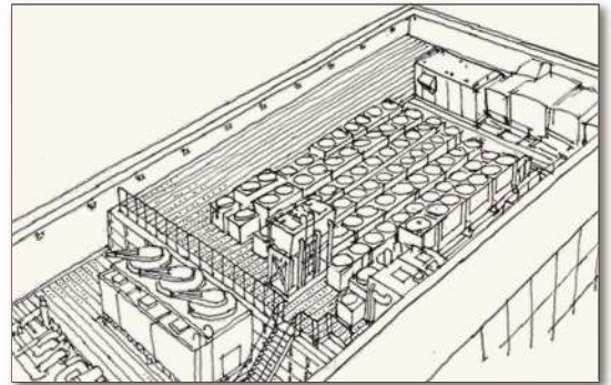
発電機用防振免震装置
