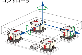
空圧アクティブ微振動ユニットとコントローラ
