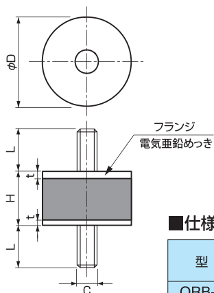
■寸法図 (単位mm)
